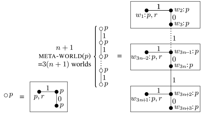
Fig. 11: META-WORLD( p )
