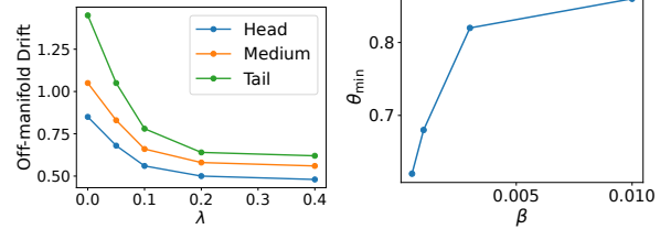
(c) Drift vs. \lambda . (d) Separation vs. \beta .
